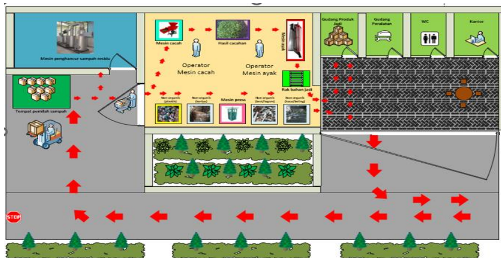
Gambar 6 . Tata Letak Fasilitas Usulan TPS3
