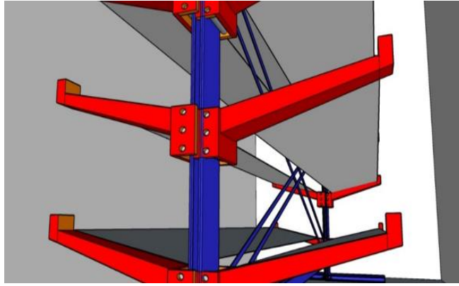
Gambar 13. Layout Usulan Gudang Peralatan
